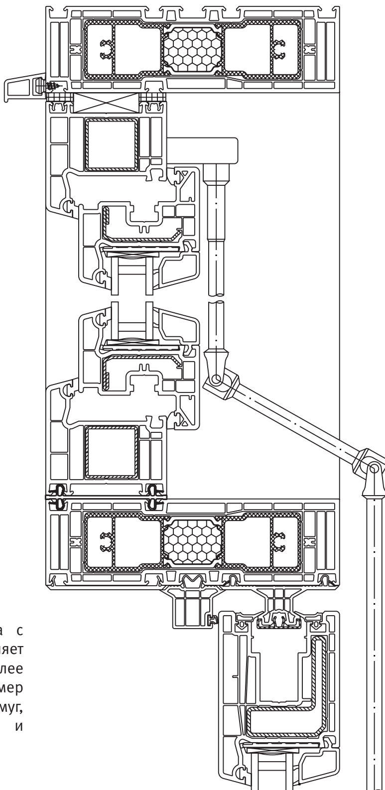
вертикальное сечение
