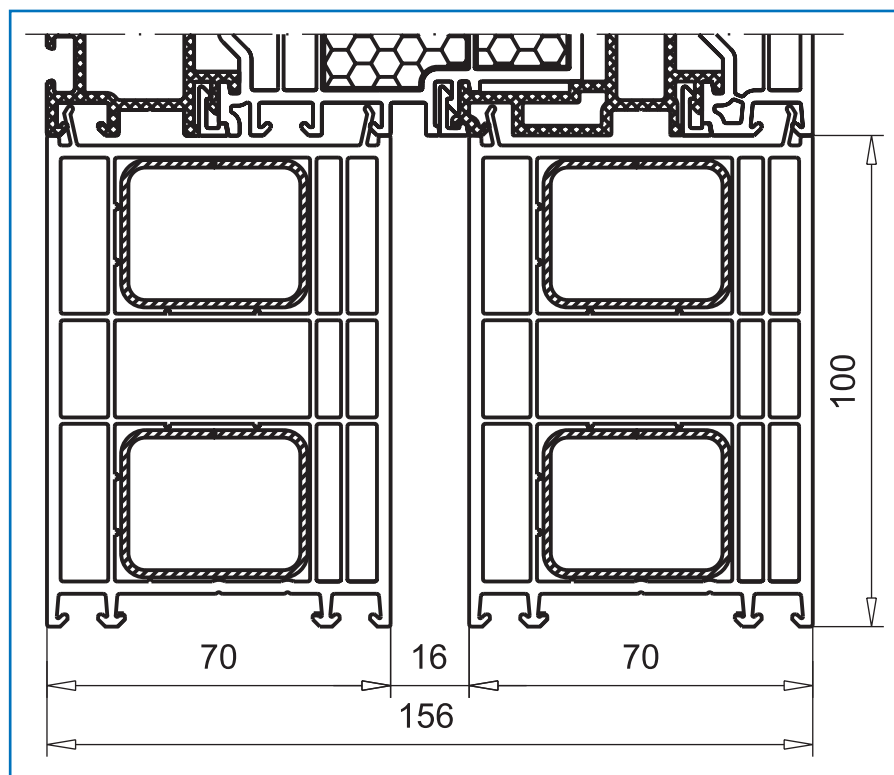
расширители SOFTLINE, установленные под порог
